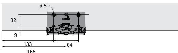
vrtání pro přední dveře levé, pravé zrcadlově
