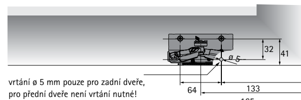
vrtání pro zadní dveře levé, pravé zrcadlově
