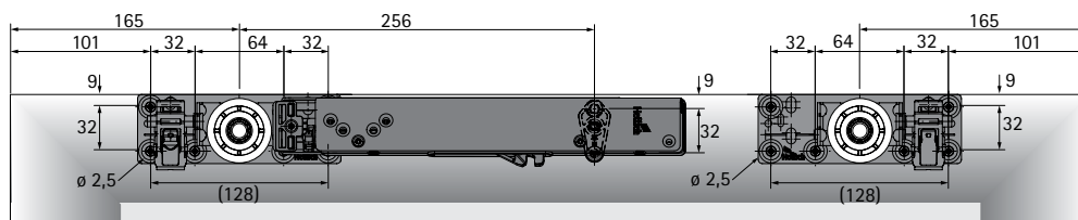
vrtání pro zadní dveře
