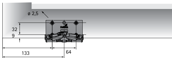
vrtání pro přední dveře levé, pravé zrcadlově
