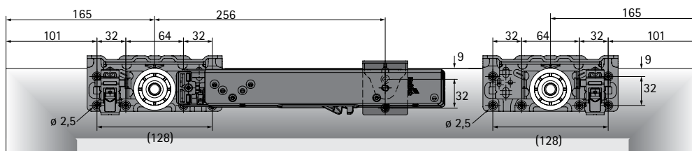
vrtání pro přední dveře levé, pravé zrcadlově
