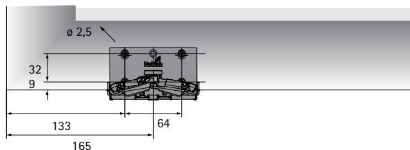
vrtání pro přední dveře levé, pravé zrcadlově
