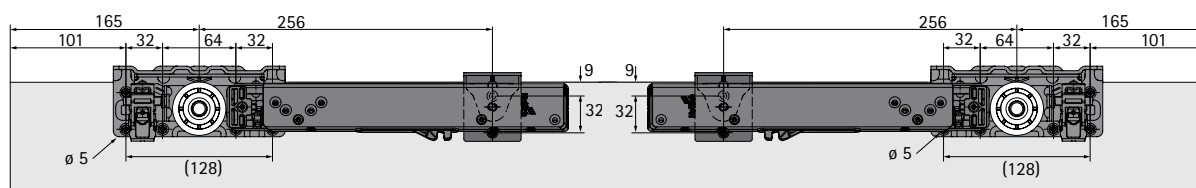
vrtání pro přední dveře
