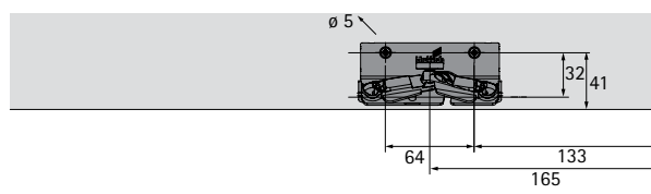
vrtání pro zadní dveře levé, pravé zrcadlově
