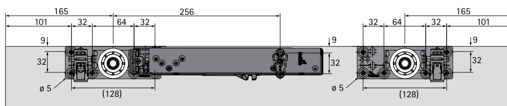
vrtání pro zadní dveře
