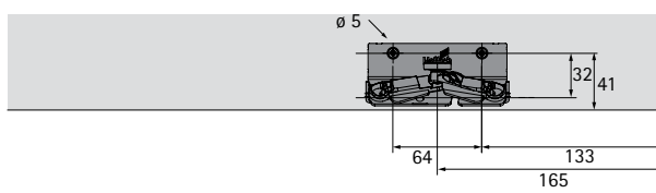
vrtání pro zadní dveře levé, pravé zrcadlově
