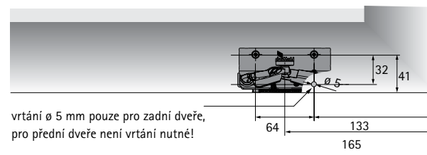
vrtání pro zadní dveře levé, pravé zrcadlově
