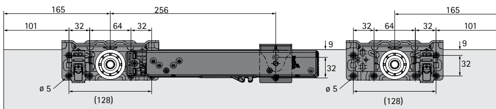
vrtání přední dveře levé, pravé zrcadlově
