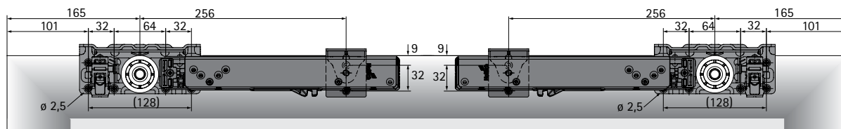
vrtání přední dveře
