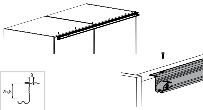
montáž horního profilu
